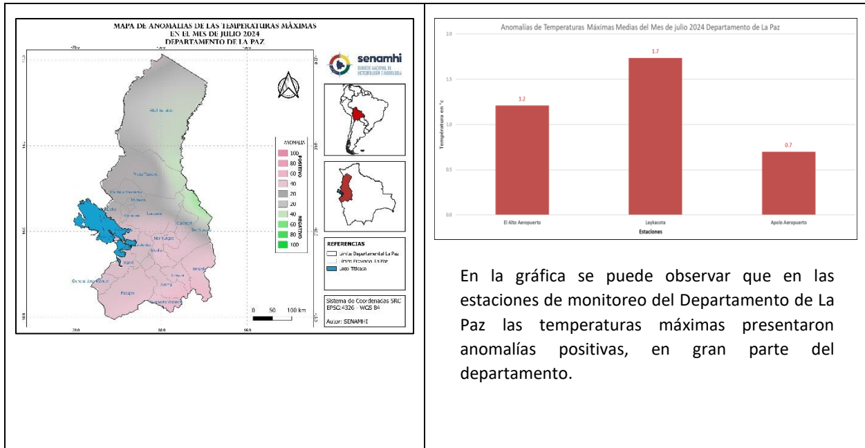
Ilustración 6 Mapa de Anomalía de Temperaturas Máximas para el mes de julio 2024
