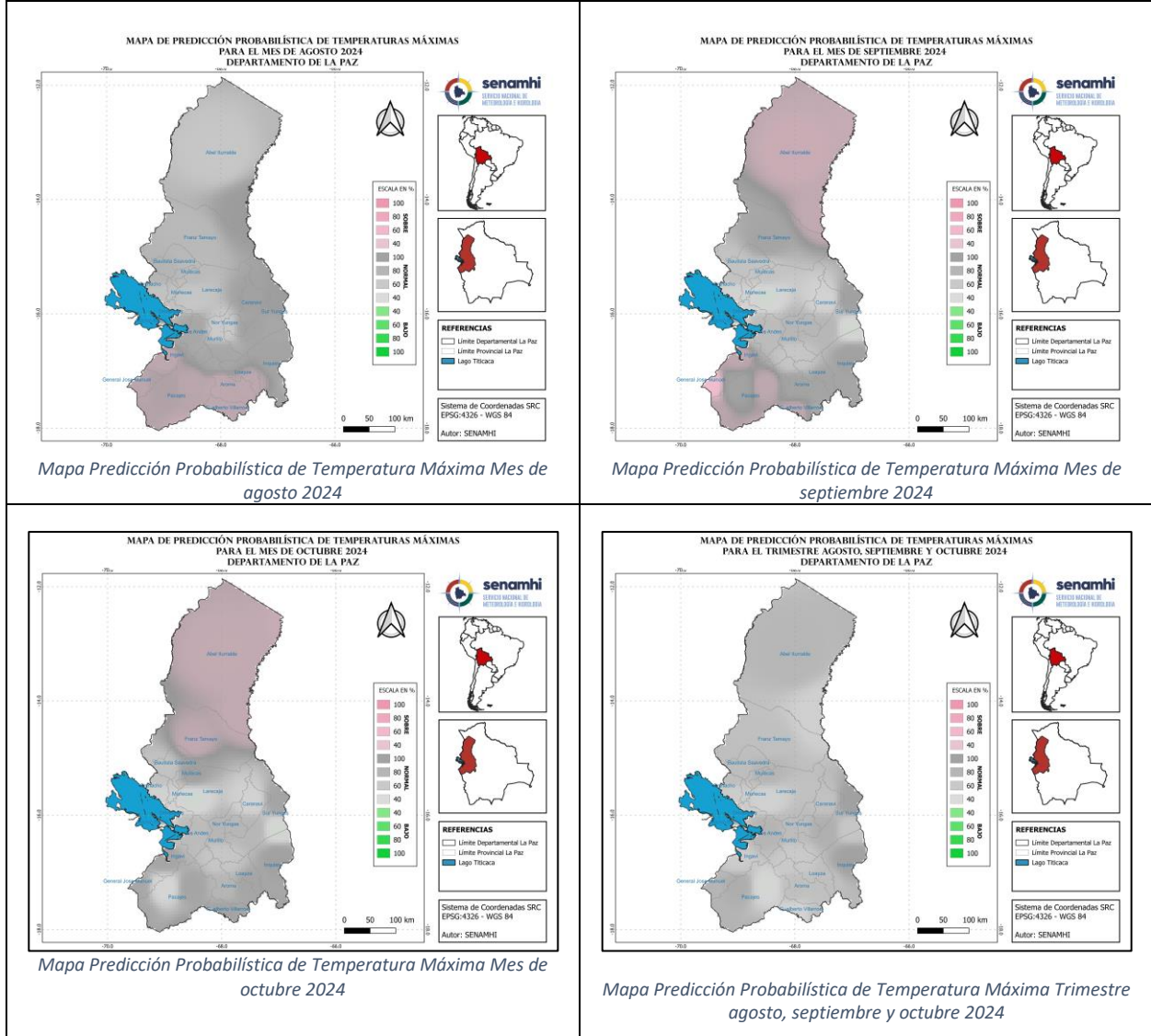
Ilustración 9 Mapas de Predicción Probabilística de las Temperaturas Máximas Medias para el trimestre ASO 2024
