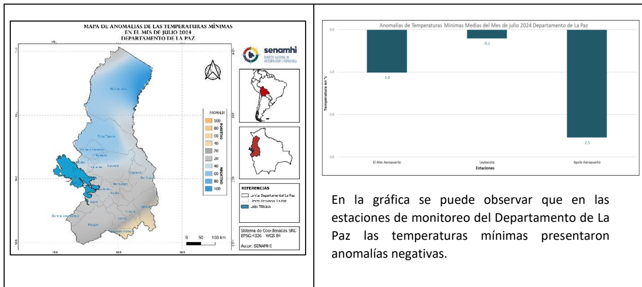
Ilustración 7 Mapa de Anomalia de Temperaturas Mínimas para el mes de julio 2024
